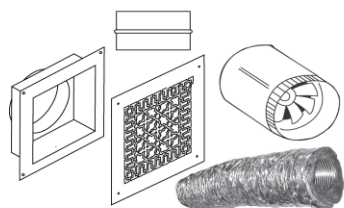
FO-HD - Sortie d'air chaud complémentaire
