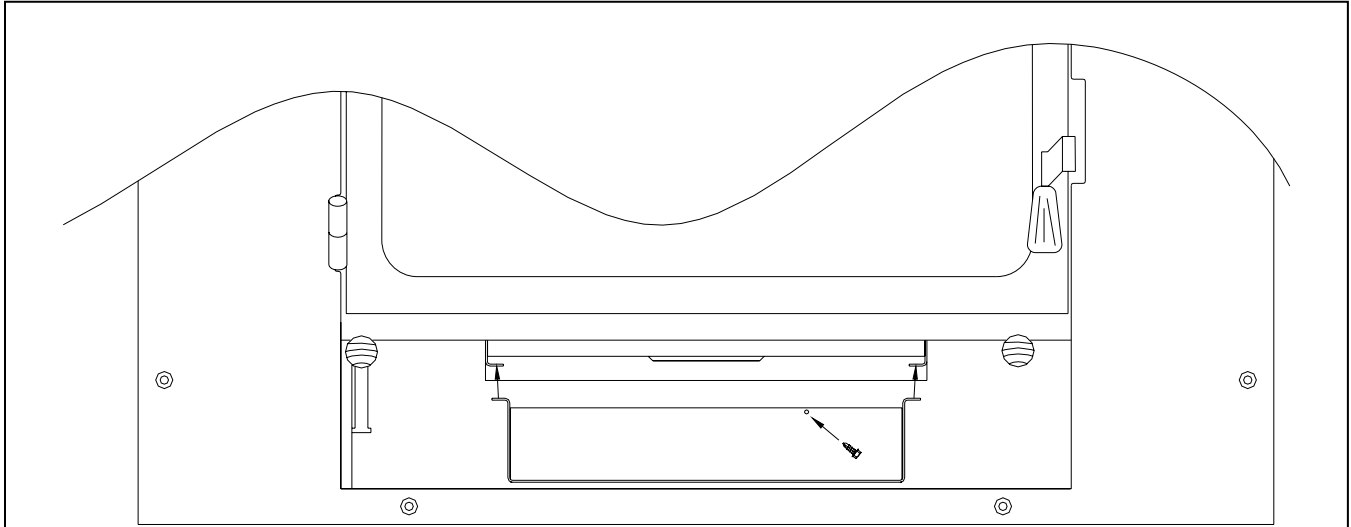
Figure 1 Installation du support pour le tiroir à cendres / Ash pan support installation
